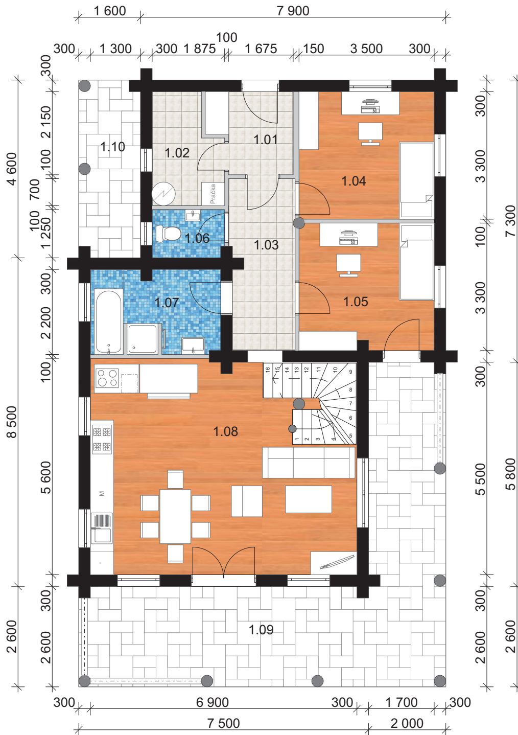
Tabulka místností 1.NP
